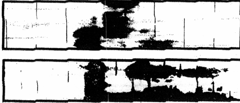
Şəkil. /fa:mi:je/ və /di:fi:tsjel/ sözlərinin spektroqramları
