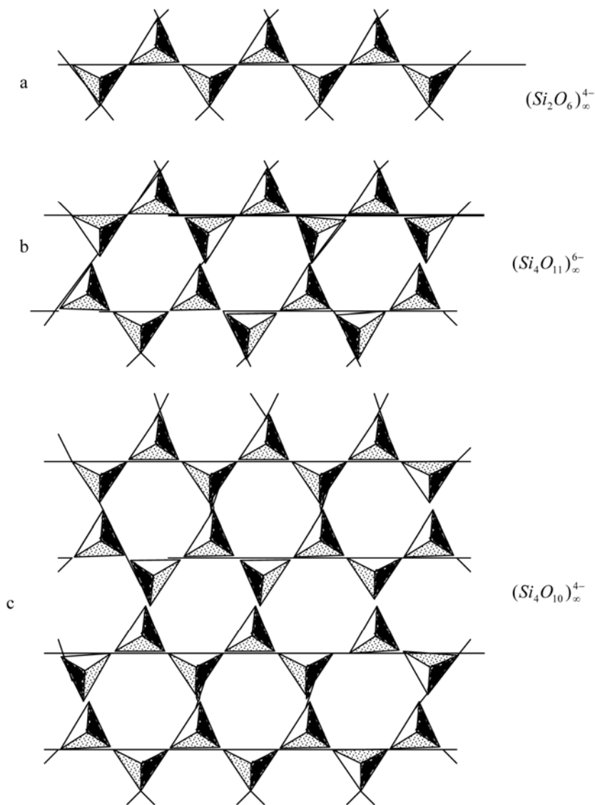
Şəkil 5. Silisium oksigen radikallar:- a- zəncirvari; b – lentşəkilli; c - vərəqşəkilli
