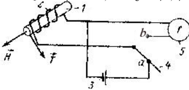
Şəkil 38. Proton maqnitometrin prinsipial sxemi.
