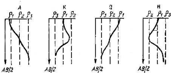
Şəkil.67. Üç laylı ŞEZ əyrisinin tipləri.
