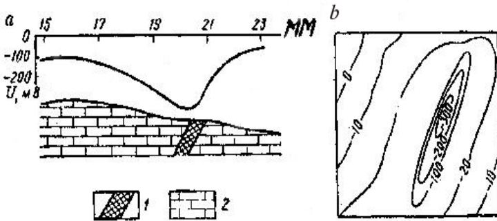
Şəkil.71. Potensial üsulu ilə müşahidə sxemi (a) gradient potensialı (b) ÖC ölçmə cihazı.
