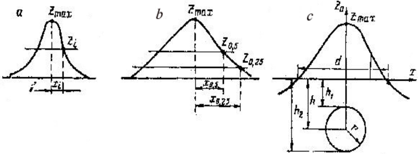
Şəkil 40. Z-əyriyələri; a-küçük qalınlıqlı laylar üzərində; b-qalın laylar üzərində; v-kürə üzərində.
