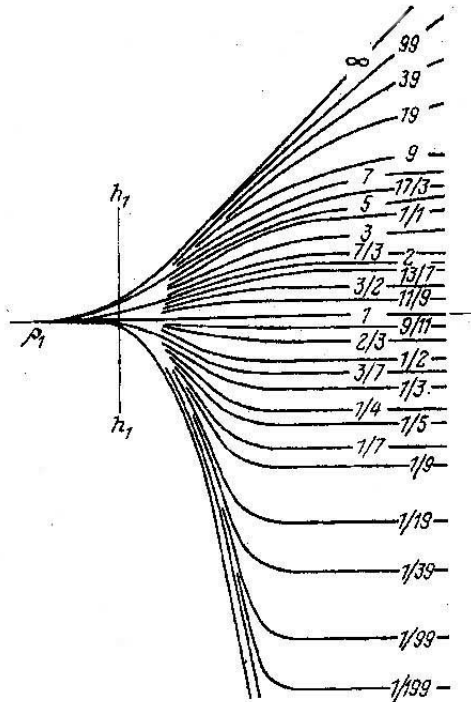
Şək.68. İkilyalı \rho_2 paletkası.
