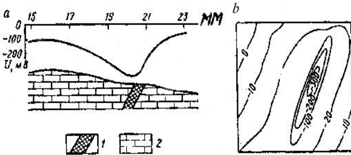
Şəkil.72 Təbii sahə üsulu ilə aparılan işin nəticələri. a- Tərkibində müxtəlif metallar olan damarlar üzərində sahə qrafiki. b- Damar üzərində bərabər potensiallı izoxətlərin planı.1. Tərkibində müxtəlif metallar olan damar. 2. Damarları özündə yerləşdirən mühit.
