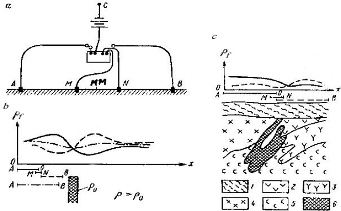
Şək. 61. Kombinasional profilləmə qurğusu (a); kiçik qalınlıqlı sərt bucaq altında düşən layın (KEP) qrafikası (b); miskoşçedan yatağı (v). 1-müasir çöküntülər, 2- Porfirit, 3-porfir, 4xloritləşmiş süxurlar, 5-istiqaətli qurğu BMNS).
