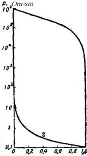
Şəkil 3. Şar formalı qoşulmalı aqreقاتların xüsusi müqaviməti 1-qoşmanın müqavimətinin, süxuru özündə yerləşdirən süxurun müqavimətinə olan nisbəti 10^{-1}/10^6 ; 2-həmçinin 10^6/10^{-1}
