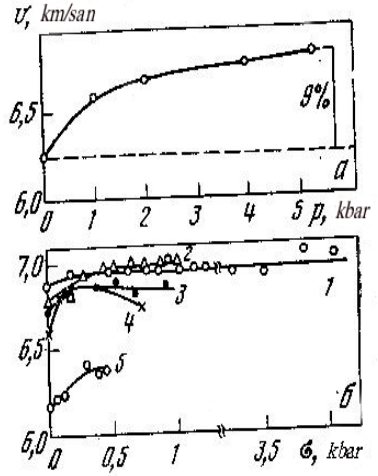
Şəkil.20. Süxurlardan hazırlanmış nümunələrdə deformasiyanın müxtəlif mərhələləri a-xətti deformasiyanın; b-həcmi deformasiyanın gərginlikdən asıllığı.
