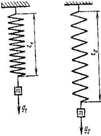
Şəkil 47. Yaylı qravimetrin sxemi.
