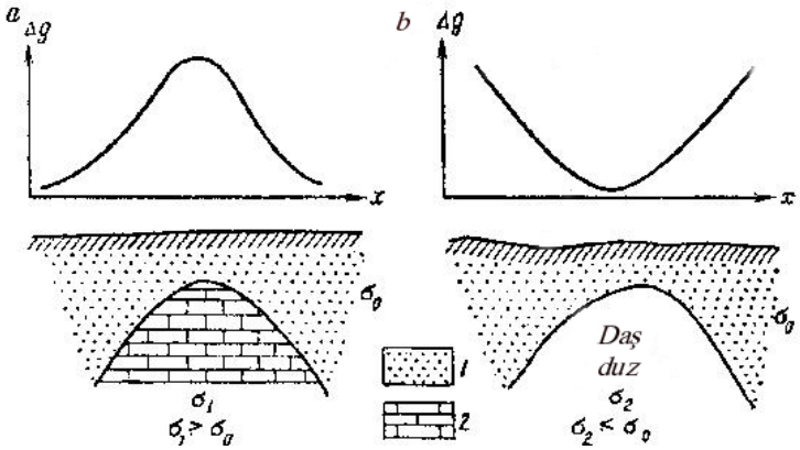
Şəkil 41. Qravitasiya anomaliyasına misal. Artıq kütlə; a-müsbət, b-mənfi 1-qum dənəcikli gilli süxur 2-əhəng daşları.
