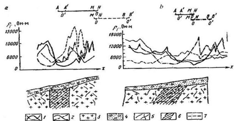
Şək. 62. Dipol profiləmənin köməyi ilə qırılmalarla əlaqədar olan çatlarla səciyyələnən ərazinin yerləşdiyi şəraitin təyini şaquli istiqamətdə (a) və sərt düşən qırılmalar üçün misal (b).
