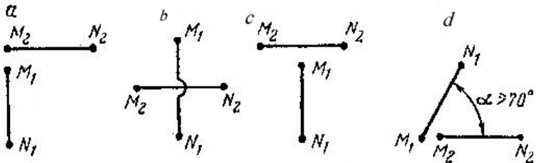
Şəkil 76. Tellurik cərəyan üsulunun ölçmə qurğuları a-Q şəkilli, b-Xaç şəkilli, v-T şəkilli, q-Bucaq şəkilli.
