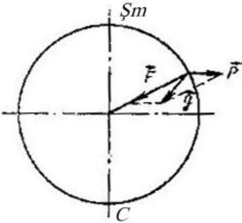
Şəkil.42. Yerin ağırlıq qüvvəsi vektoru və onun toplananları.
