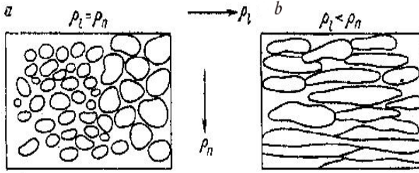
Şək. 54. Xüsusi elektrik müqavimətinin süxurun teksturasından asılılığı. Süxurlar a. bircinsli; v. qeyri-bircinsli.
