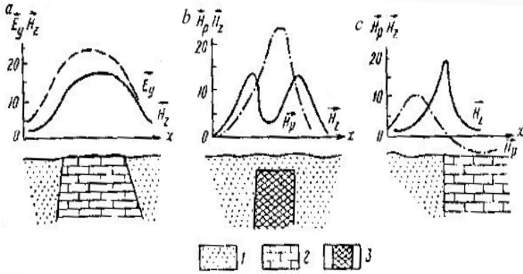
Şək.77. Radiokip üsulu ilə aparılan işlərin nəticələri. 1- gilli qum daşığı; 2- əhəng daşığı; 3-keçirici mühit.
