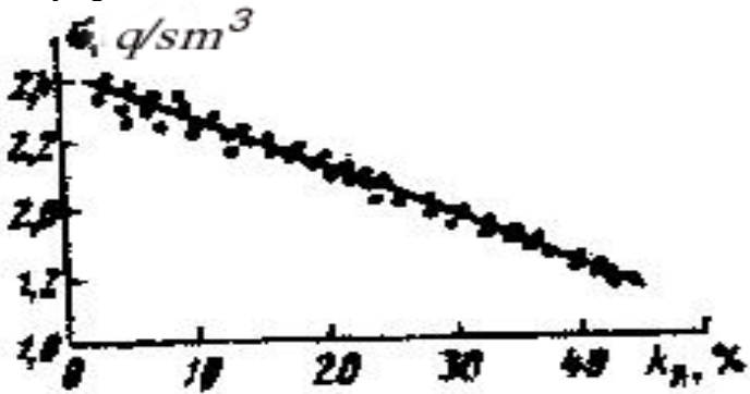
Şəkil 44. Çökmə süxurlarının sıxlığının \sigma onun məsaməliliyindən K_m asıllığı.
