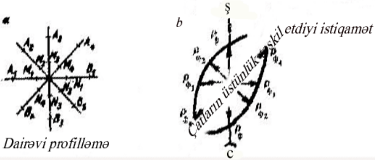
Şəkil 60 Dairəvi profilləmə.
