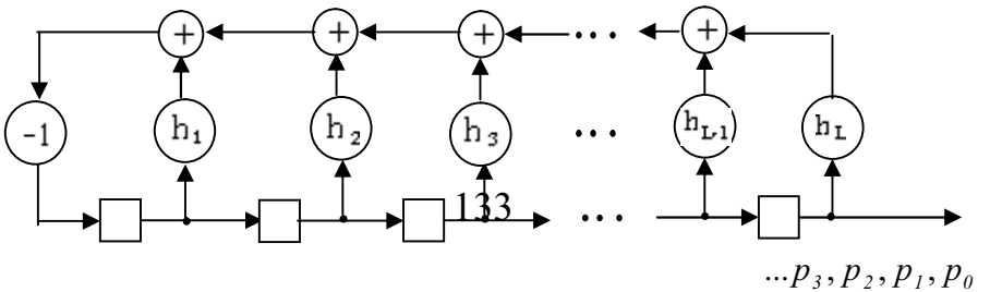
Şəkil 6. Çoxhədlilərin dövrə sürüşdürməsi qurğusu.
